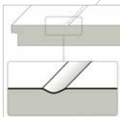
Detail Rillenfräsung
