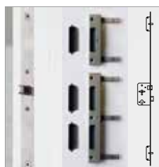
Dreifachverriegelung mit WE-Schließblech
