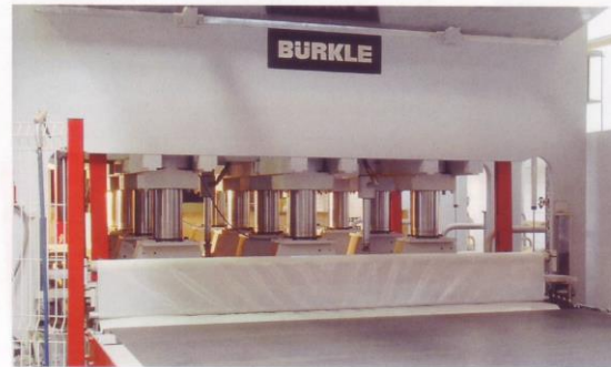
Durchlaufpresse Größe 3150 x 2350mm
